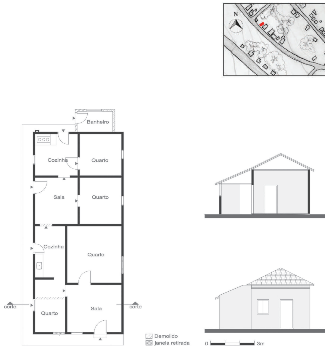
Figura 24: Planta baixa e cortes da Casa da Família Ramos.
