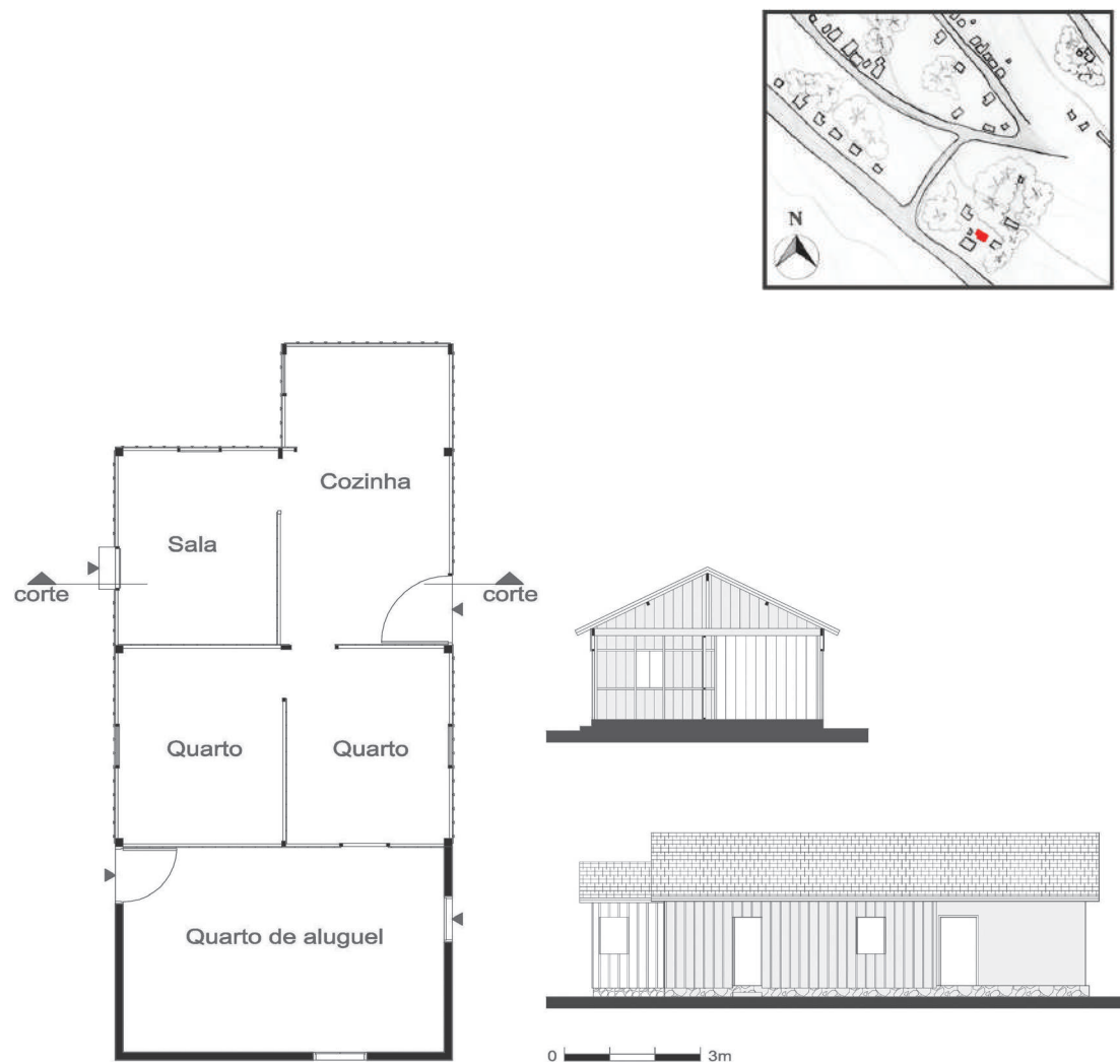
Figura 35: Planta baixa e cortes do Barraco da Gegê.
