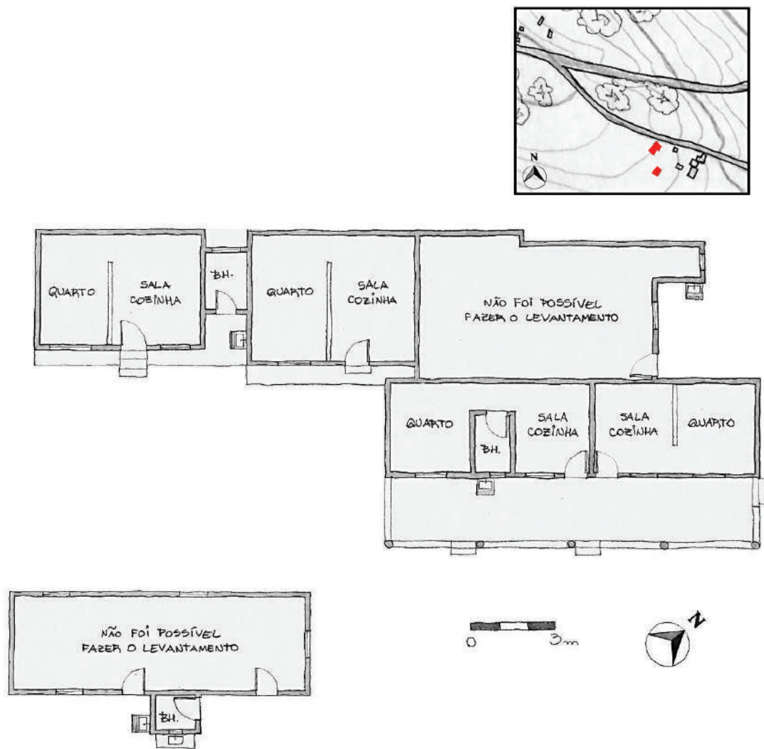
Figura 49: Planta da casa de Benedita. Parque Sabará, São Carlos. 2014.
