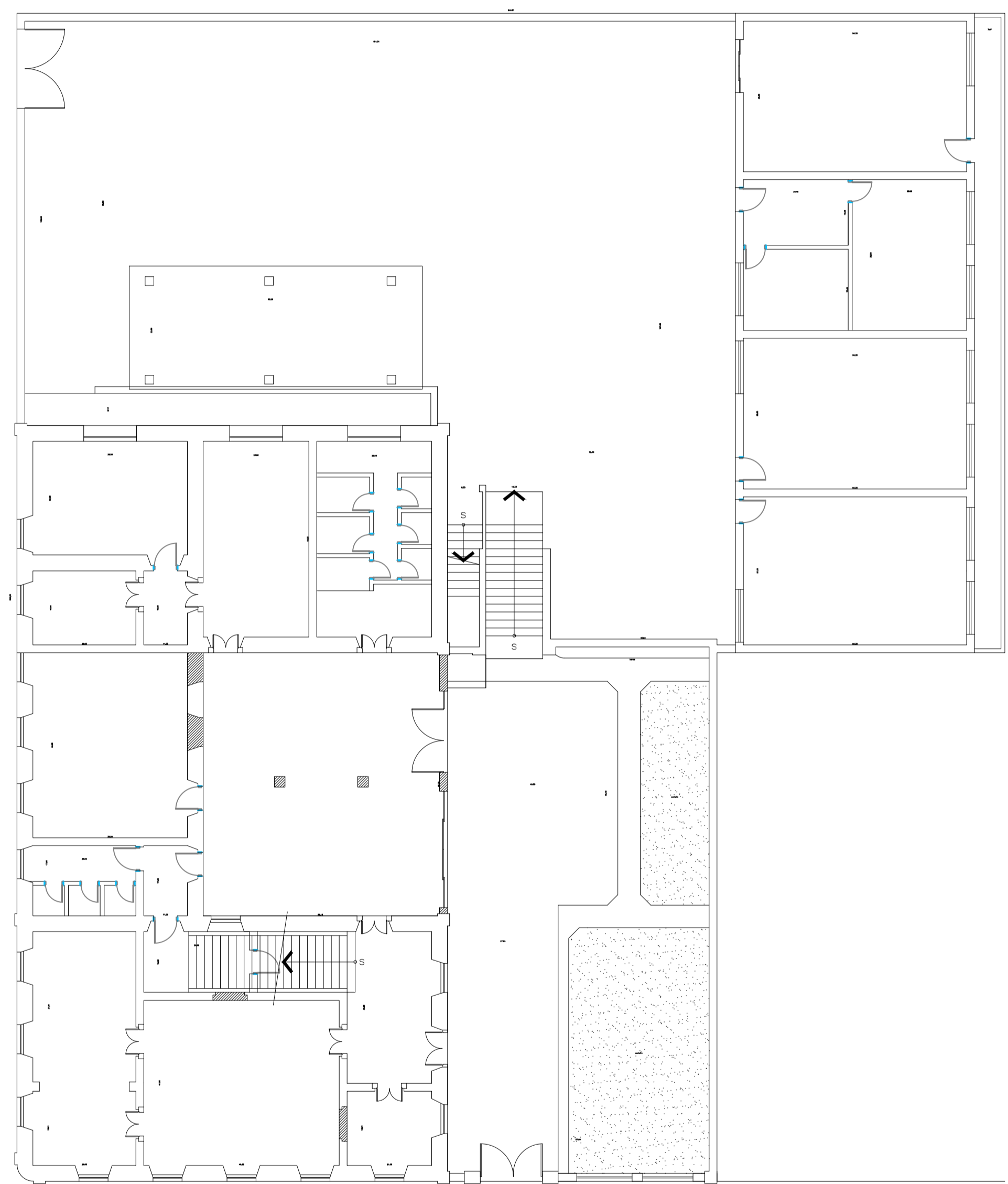
Planta térreo
